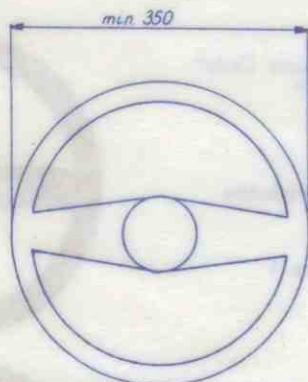
Pomiar średnicy zewnętrznej
